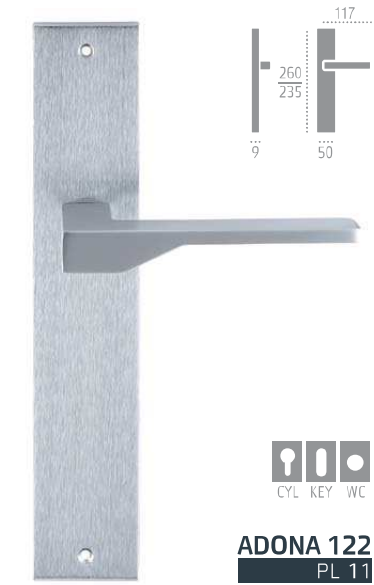
F 04 полированный хром
