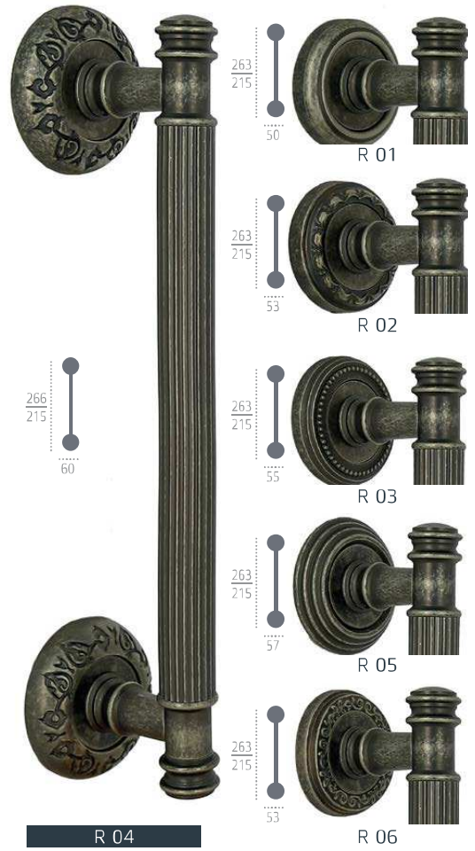
R 04 F 45 античное серебро
