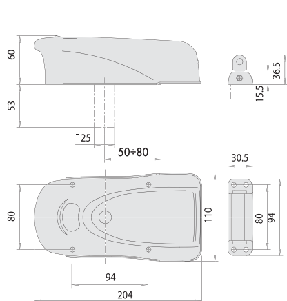
Модель 1A630
