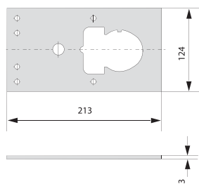
Монтажная пластина 06.429.05.0
