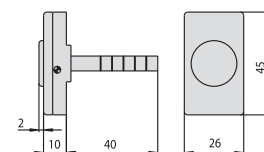
Кнопки 06.110.10.0 06.110.00.0
