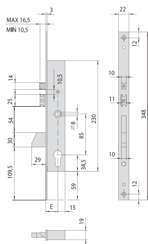
Модель 16.215
