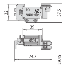
Катушка арт. 07.025.00.0
