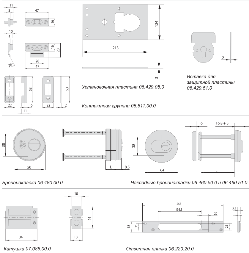
Модель 15.535
