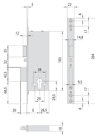
Модель 12.011
